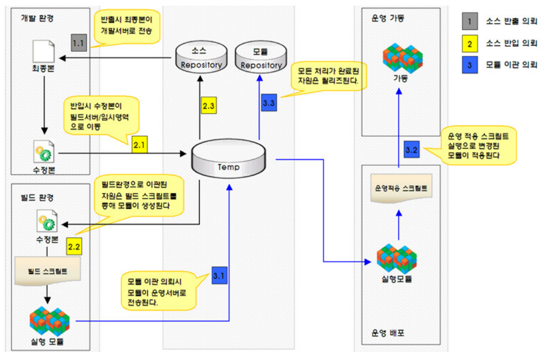
[그림 4-1] 운영환경에서의 애플리케이션 빌드·배포환경 (예시)
